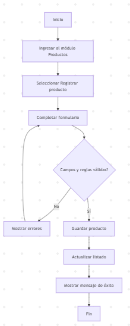
Figura 3. Diagrama de actividades del módulo de productos
