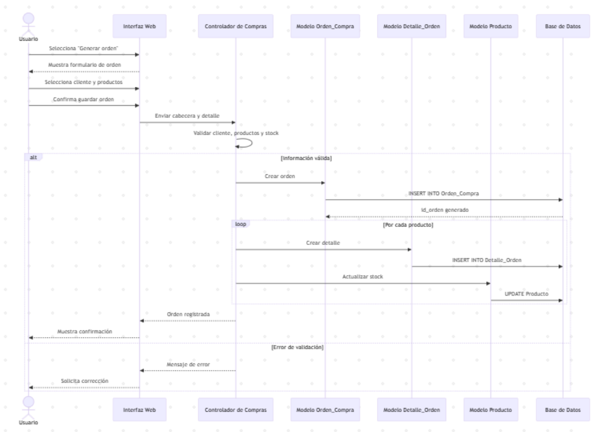
Figura 2. Diagrama de secuencia del módulo de compras
