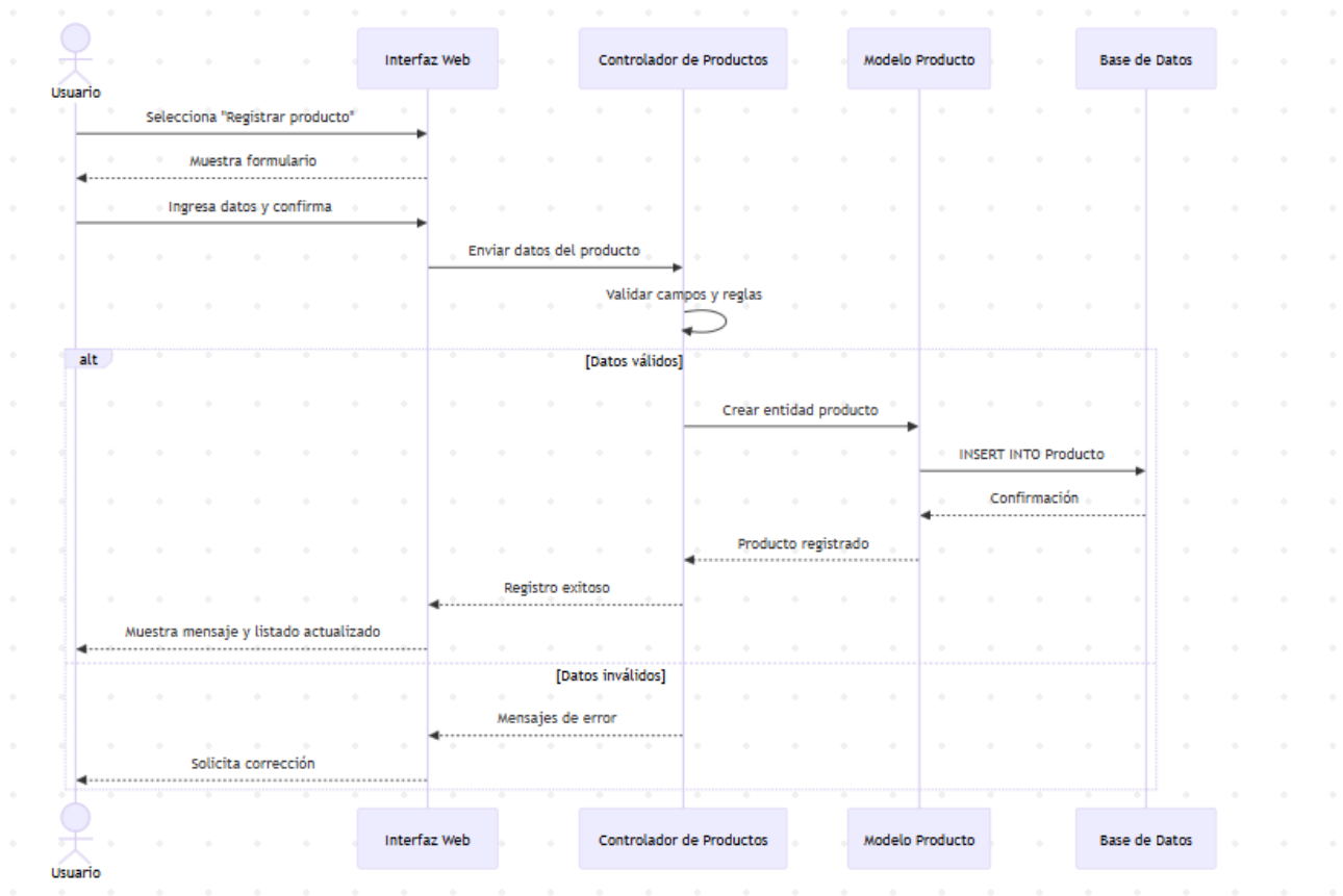
Figura 1. Diagrama de secuencia del módulo de productos
